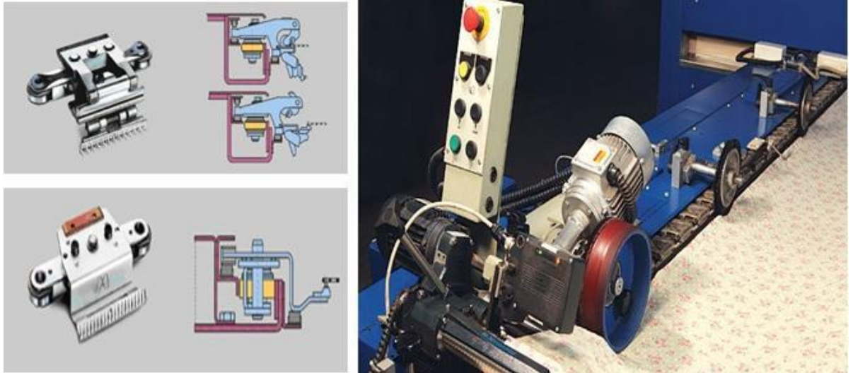
Fig.1.2 Stenter Chain
